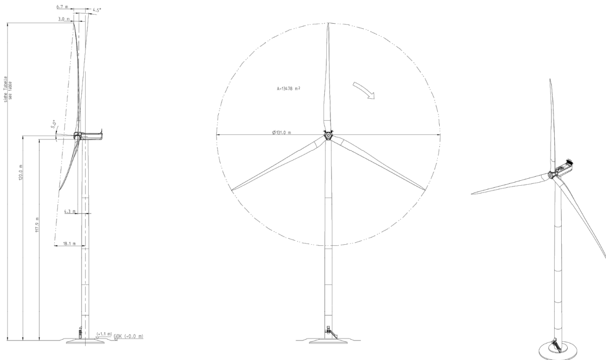
Figure 3 : vue d'ensemble de l'éolienne Nordex N131 (source : constructeur Nordex)
