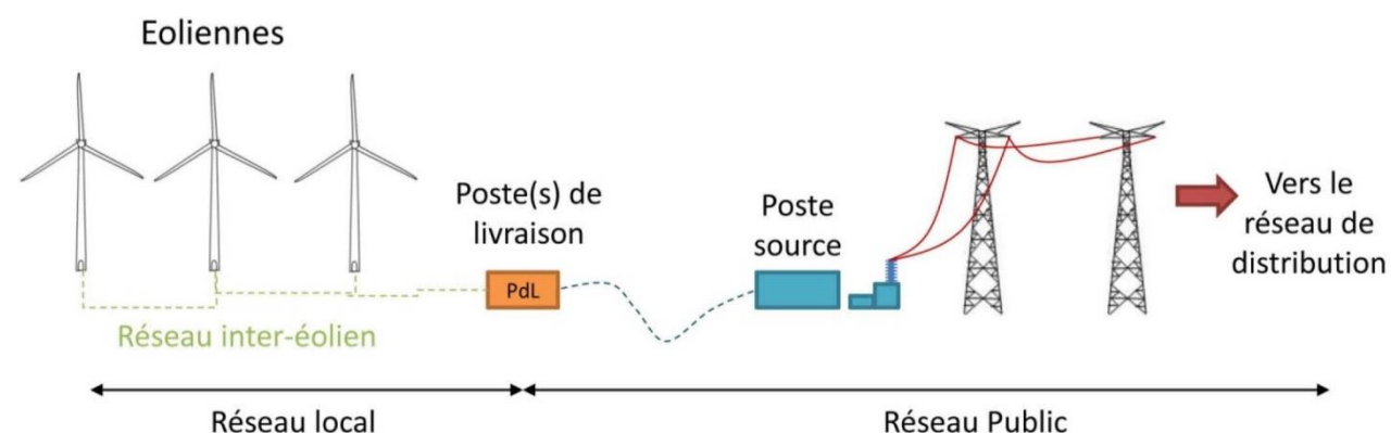
Figure 12 : Raccordement électrique des installations (source : INERIS/SER/FEE, 2012)
