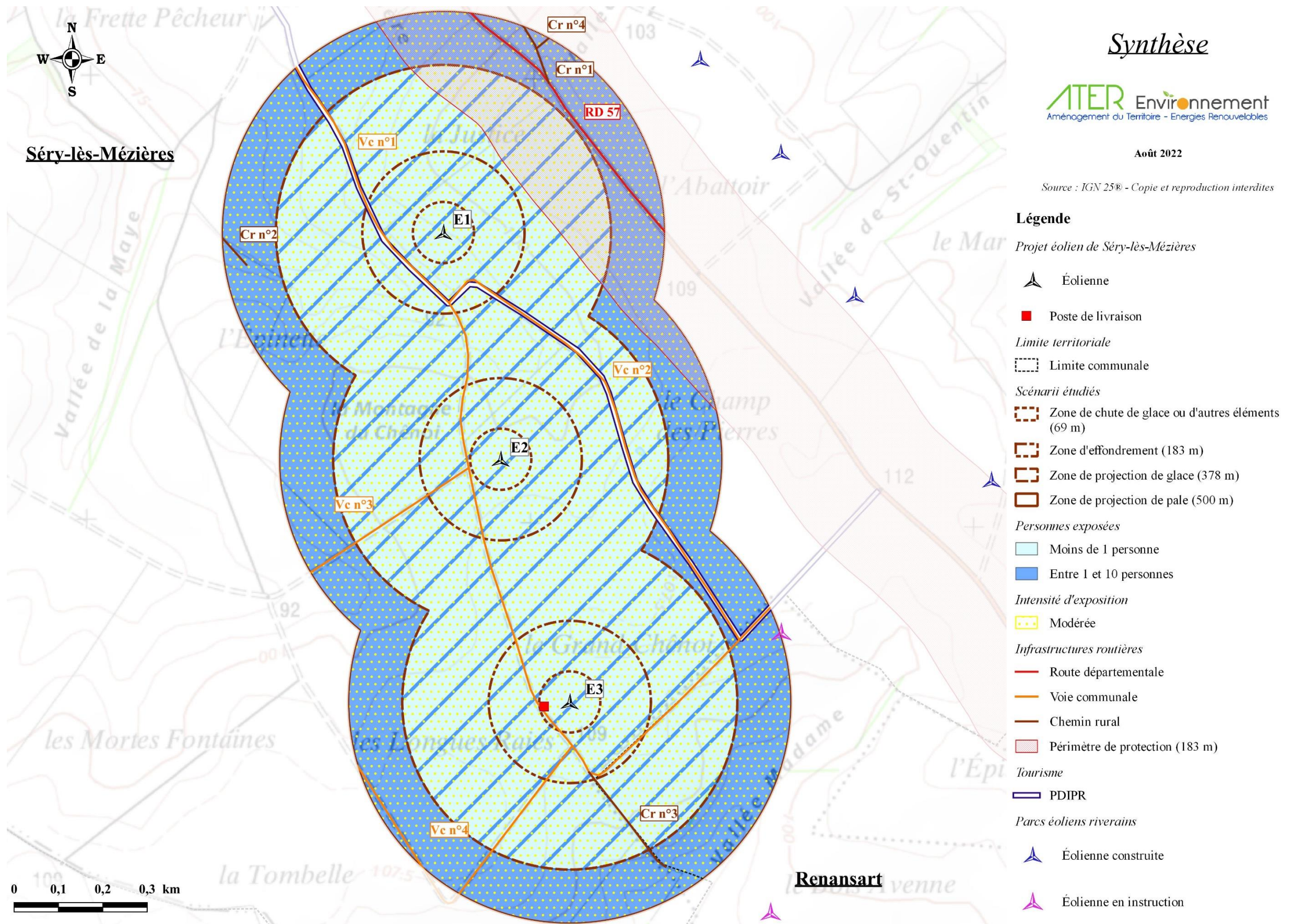
Carte 14 : Synthèse des risques dans le périmètre de dangers
