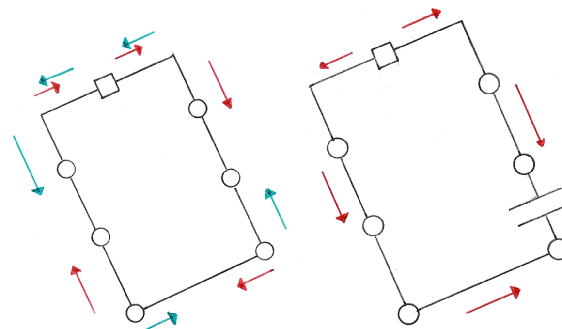
Figure 11 : Illustration du système en anneau garantissant une communication continue des éoliennes –
