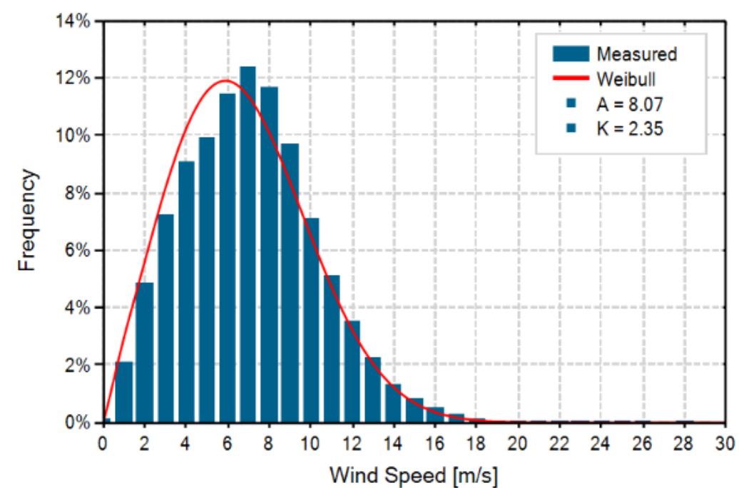
Figure 9 : Courbe de Weibull (source : VALECO, 2020)
