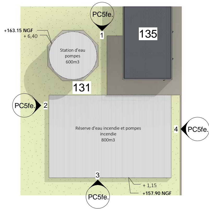
5 Plan de Toiture 1 : 500
