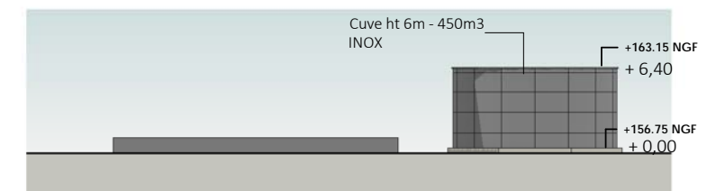
4 Façade Sud 1 : 500
