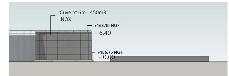
2 Façade Nord 1 : 500
