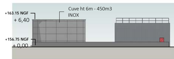
3 Façade Ouest 1 : 500
