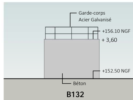
4 Façade Nord 1 : 200
