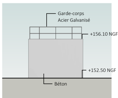
5 Façade Est B133 1 : 200
