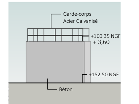
8 Façade Ouest B133 1 : 200
