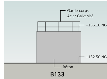
6 Façade Nord 1 : 200
