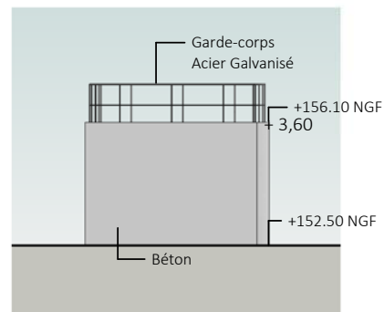
3 Façade Est B132 1 : 200
