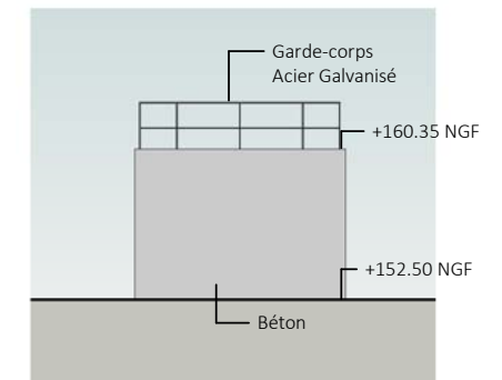
7 Façade Ouest B132 1 : 200
