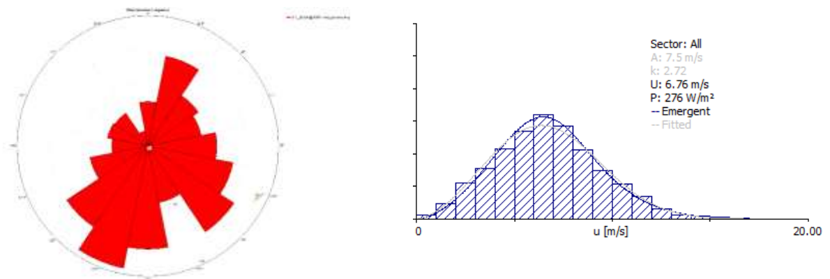
Figure 7 – Rose des vents et courbe de Weibull
