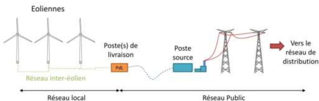
Figure 17 - Raccordement électrique des installations
