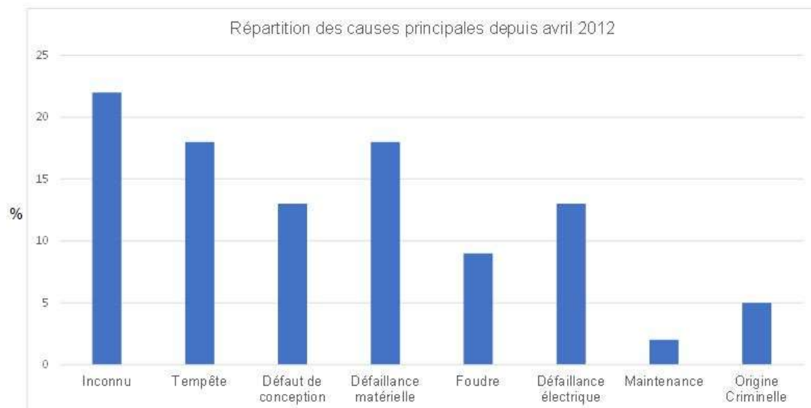
Figure 21 – Répartition des causes principales sur le parc éolien français depuis avril 2012
