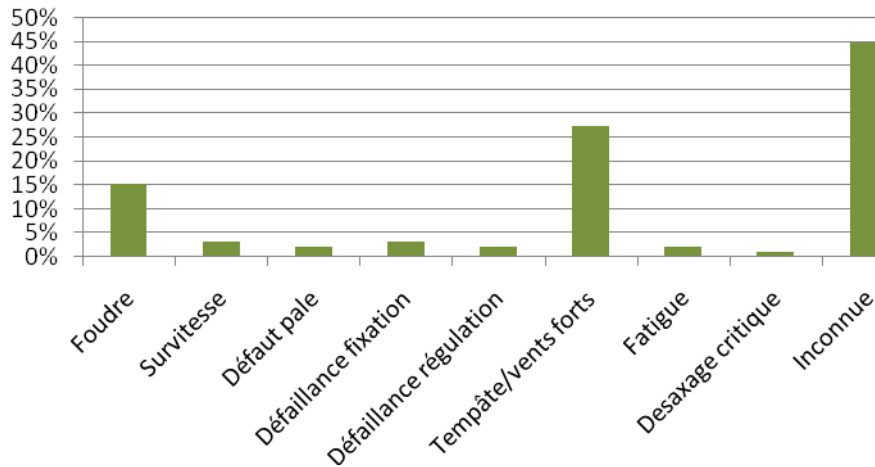
Figure 24 - Répartition des causes premières de ruptures de pales
