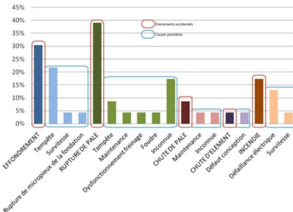
Figure 19 - Répartition des événements accidentels et de leurs causes premières sur le parc d'aérogénérateurs français entre 2000 et 2011
