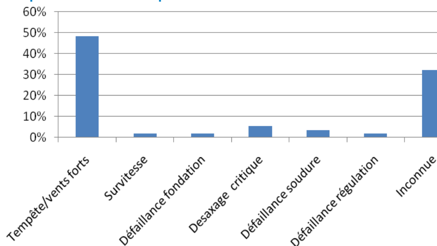
Figure 23 - Répartition des causes premières d'effondrement
