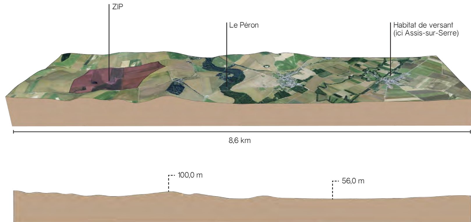
Figure 90 : Coupe de principe entre Assis-sur-Serre et le site d'implantation potentiel
