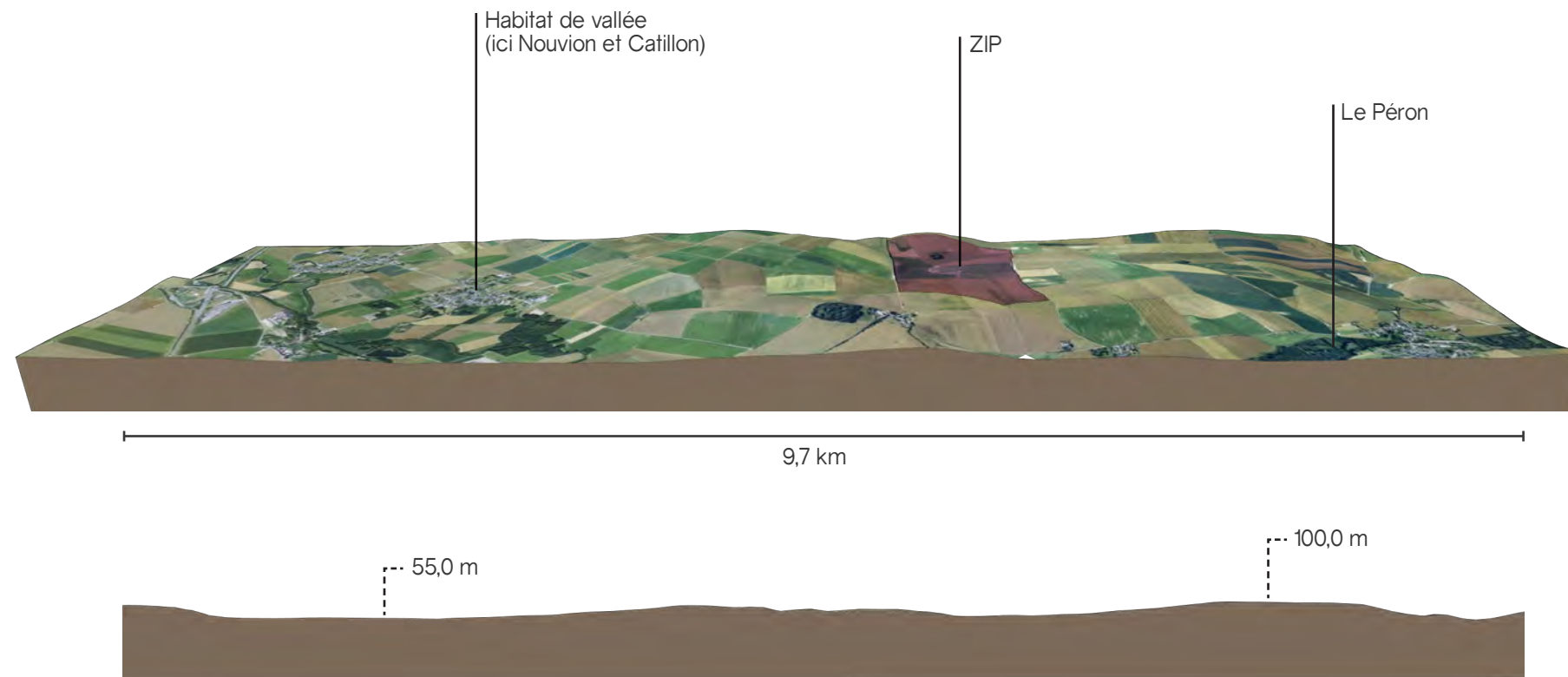
Figure 88 : Coupe de principe entre Nouvion-et-Catillon et le site d'implantation potentiel
