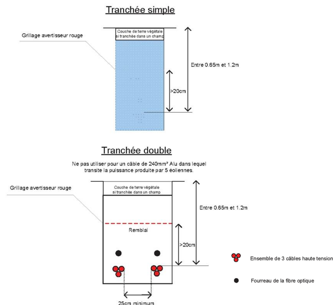
Figure 12 : Coupes-types de tranchées (source : Nordex, 2019)
