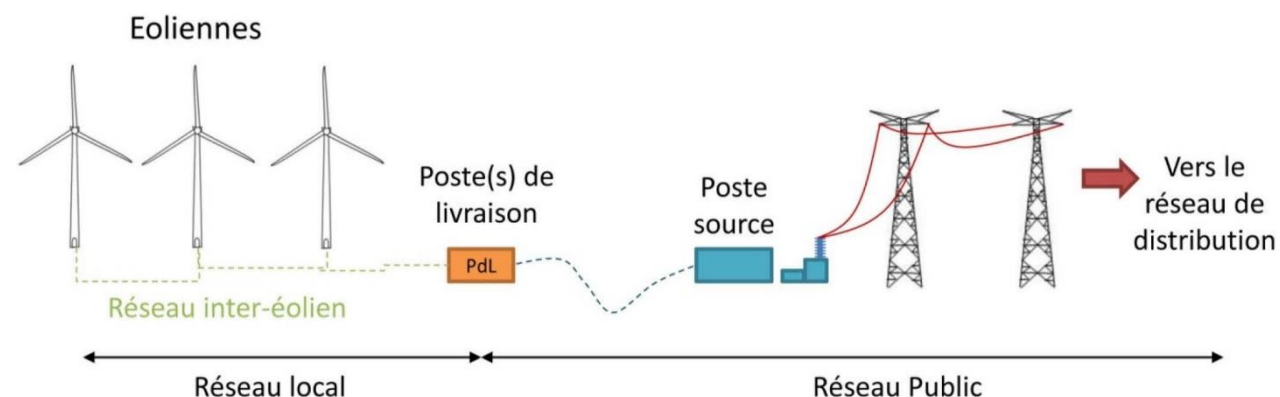
Figure 11 : Raccordement électrique des installations (source : INERIS/SER/FEE, 2012)
