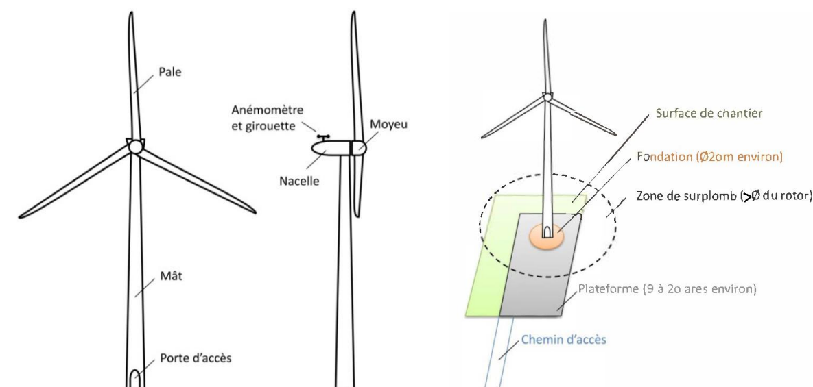
Figure 9 : Schéma simplifié d'un aérogénérateur (à gauche) - Illustration des emprises au sol d'une éolienne (à droite) (Les dimensions sont données à titre d'illustration pour une éolienne d'environ 150 m de hauteur totale) (source : Guide de l'INERIS, mai 2012)
